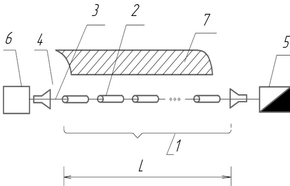
Рисунок 2 – Схема установки на основе поверхностной волны для сушки древесины
